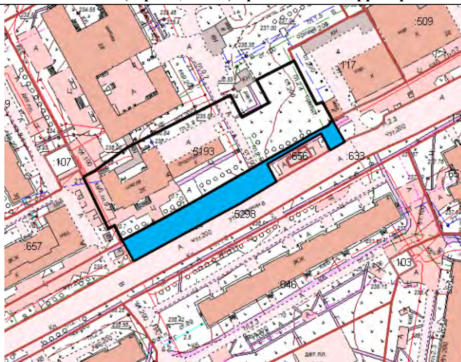
План (чертеж, схема) прилегающих территорий
