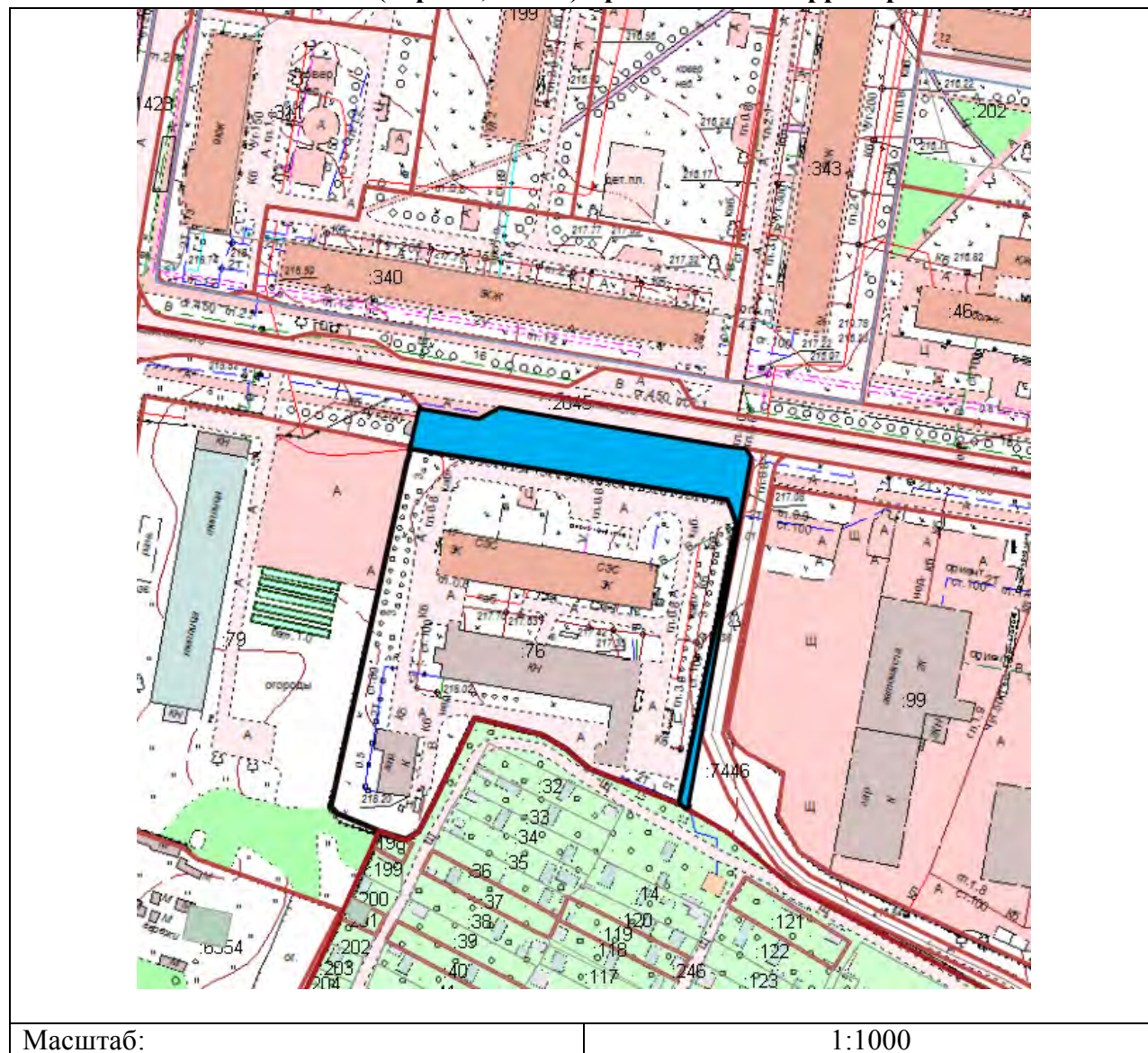
План (чертеж, схема) прилегающих территорий
